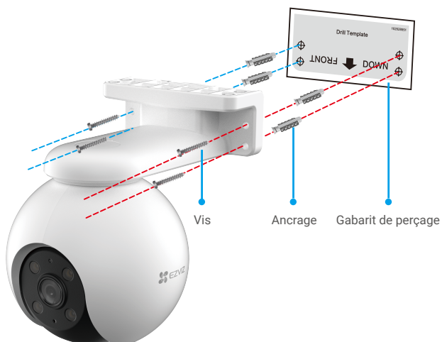
Fig. 2 Montage mural
