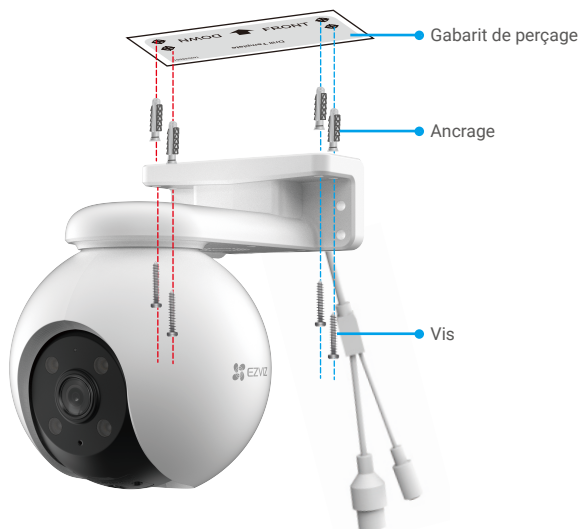
Fig. 1 Montage au plafond
